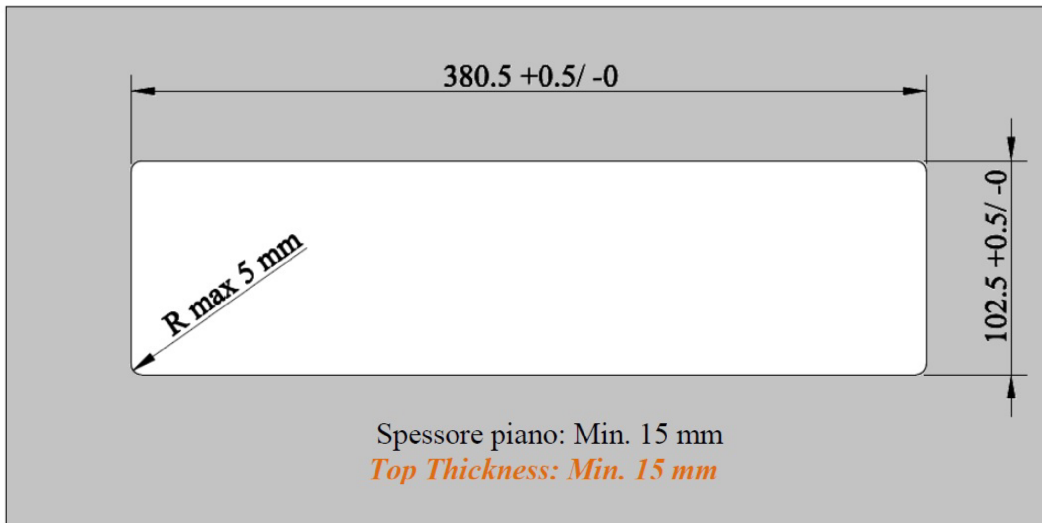
Dimensioni di montaggio(mm) Cut-out dimensions(mm)
